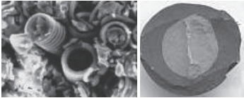
ビーズの表面の状態 (CMC が外に出ている) 破断面 (外皮がCMC含有層)
